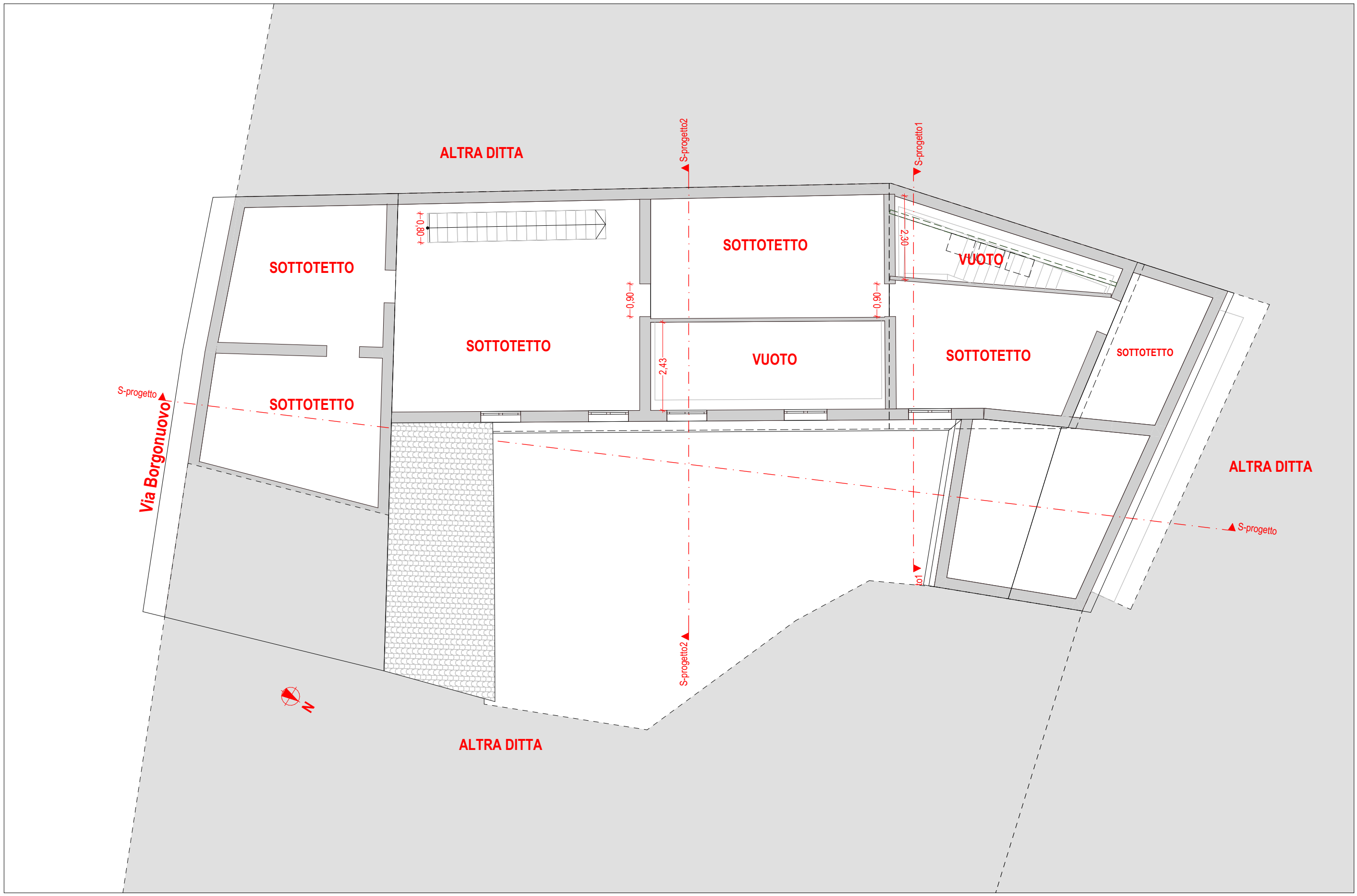
PIANO SOTTOTETTO PROGETTO
